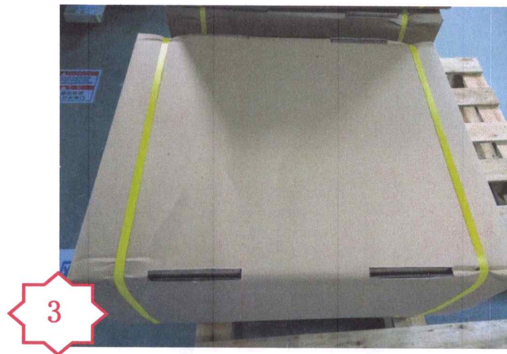
图三，确认 PA504 无漏装后，将 22 的内箱与外箱配合并打包装带待出货
